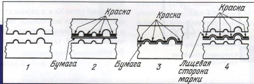
Схема конгревного тиснения (по Н. Владинцу)
